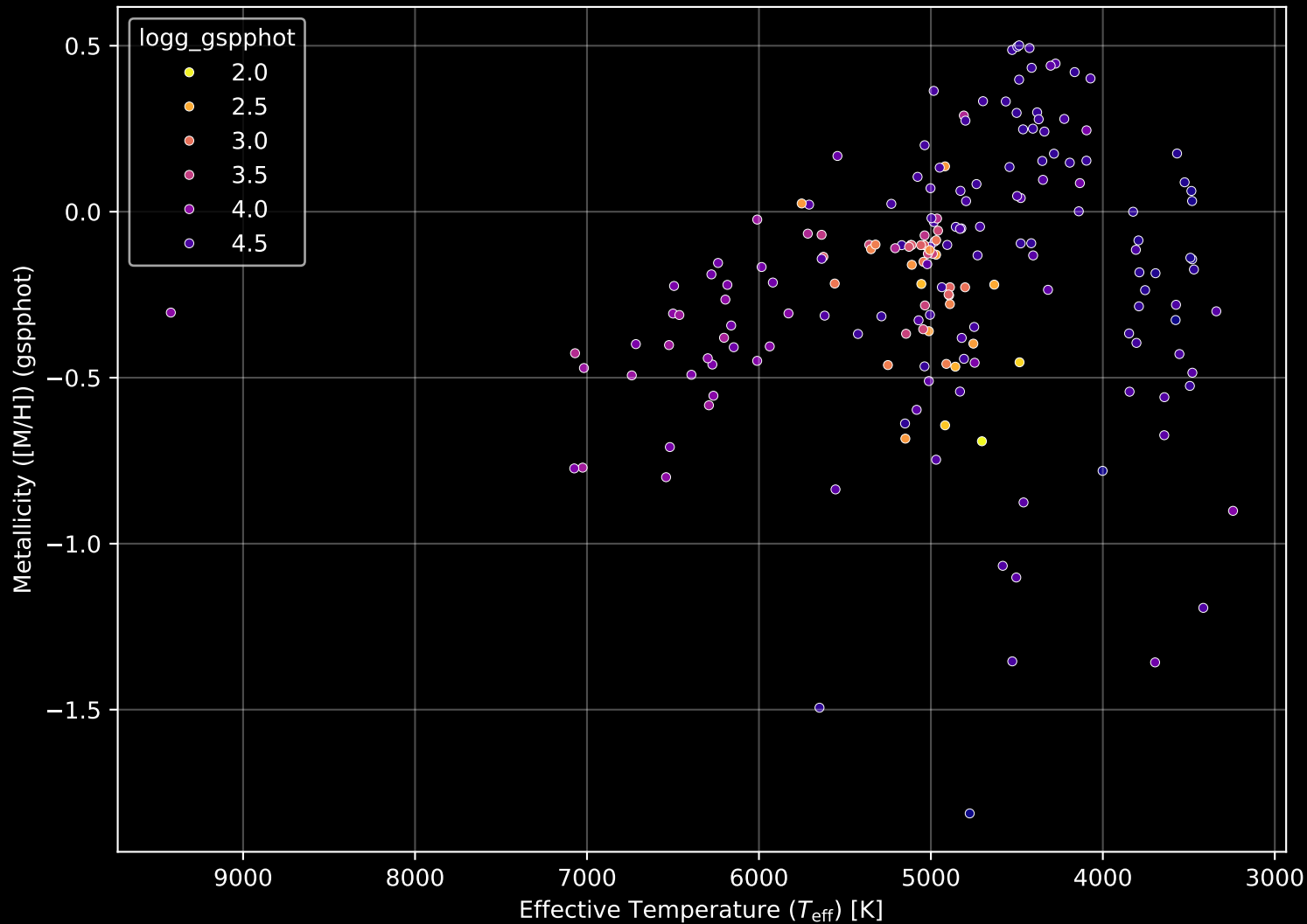
APOGEE DR17 Field: [160+60] Stellar Population Parameters (n= 187)
